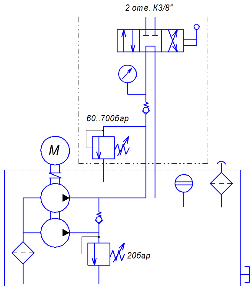
Рис.2 (Гидравлическая схема)
