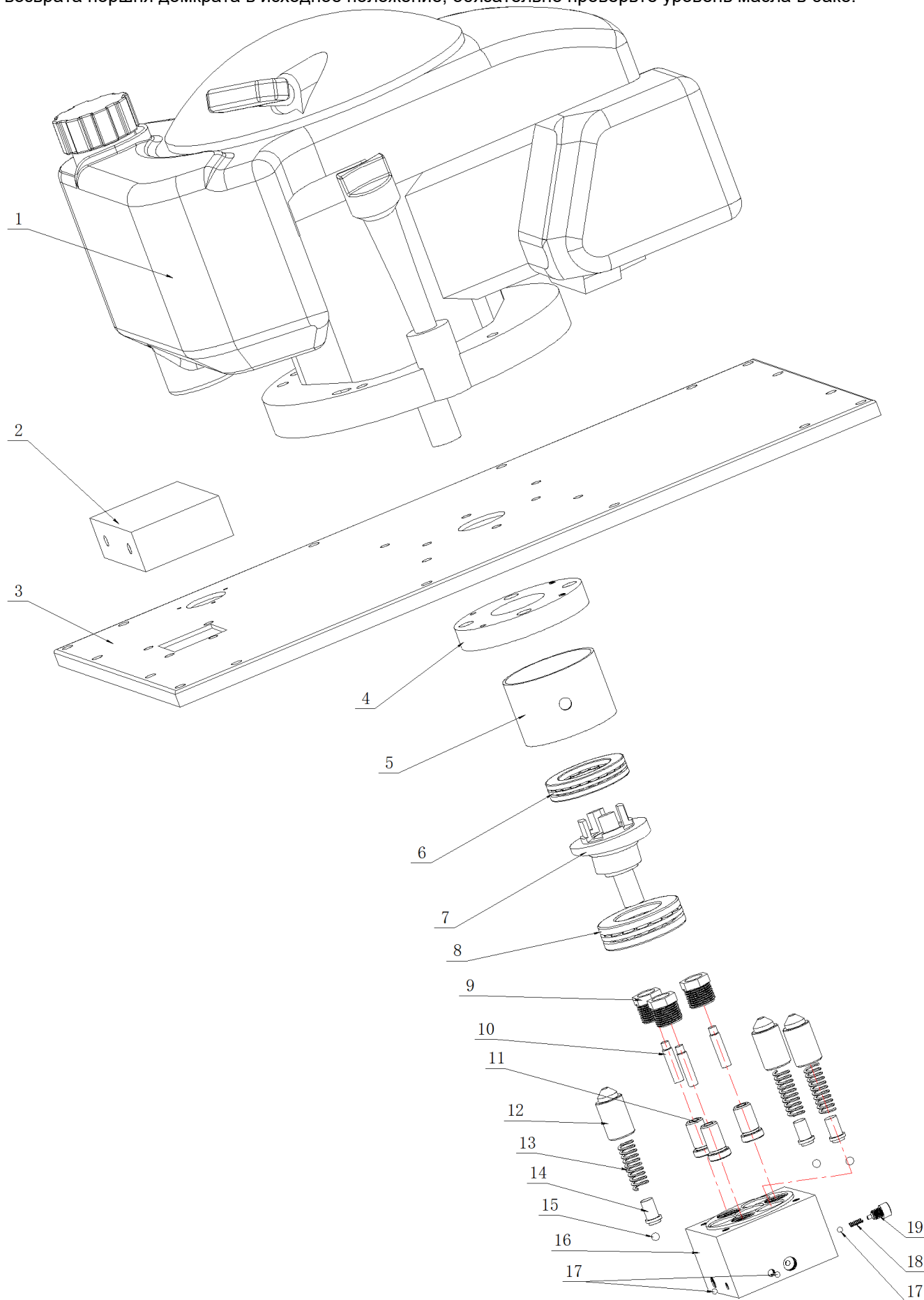
Рис.3 (Взрыв-схема)
